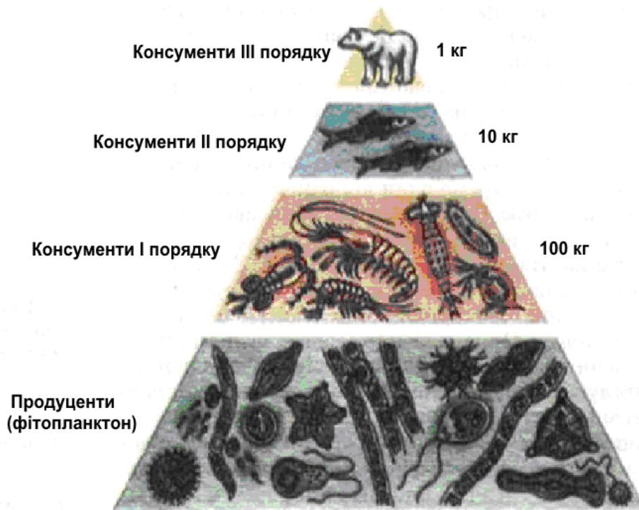
Мал.13. Екологічна піраміда.
