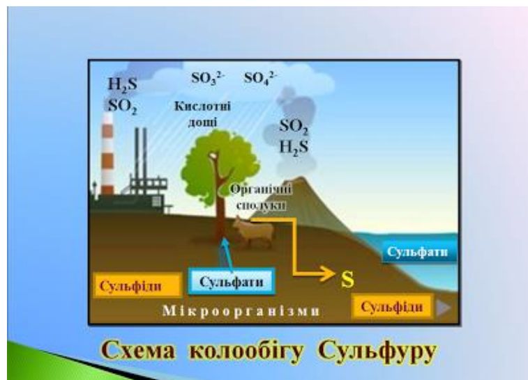
Мал.7. Кругообіг сульфуру.
