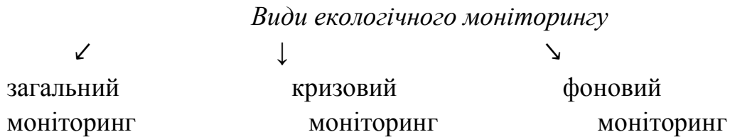
Рис. 10. Види екологічного моніторингу
