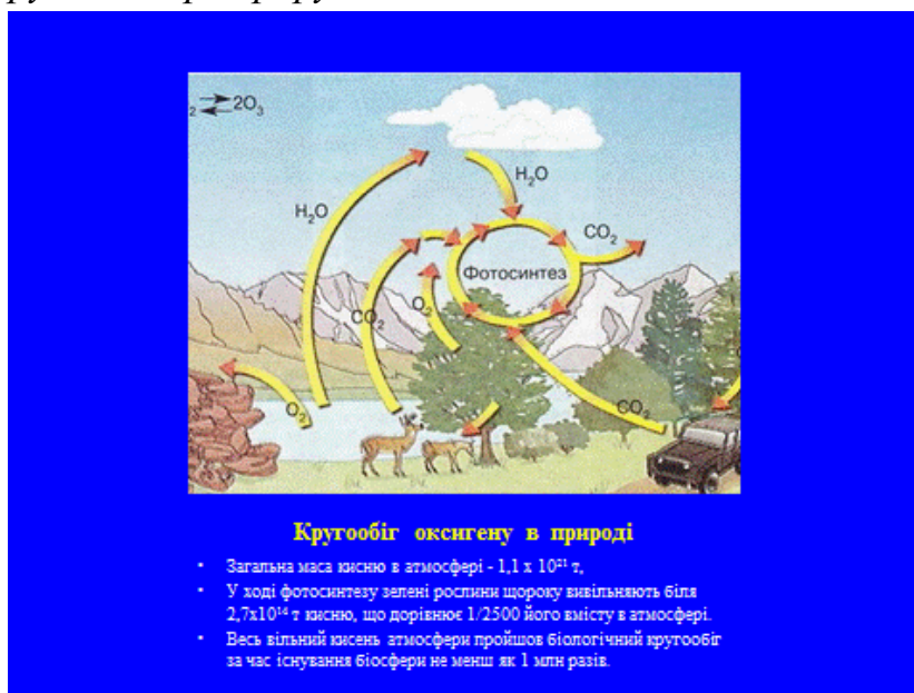
Мал.9. Кругообіг кисню.
