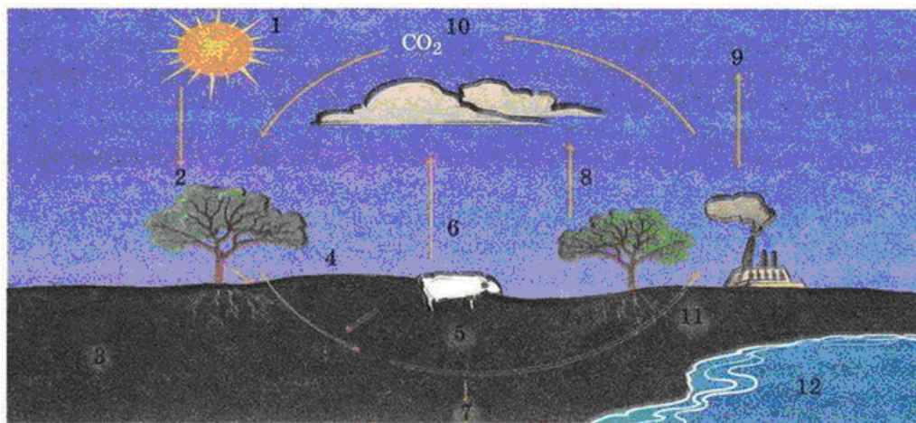
Колообіг Карбону у природі: 1. Сонячне світло. 2. Фотосинтез. 3. Гниття. 4. Органічні речовини рослинного походження. 5. Тваринні рештки і продукти гниття. 6. Дихання тварин. 7. Ґрунти і торф. 8. Дихання рослин. 9. Транспортні й промислові викиди. 10. Цикл карбон(IV) оксиду. 11. Кореневе дихання. 12. Карбоновмісні речовини океану
