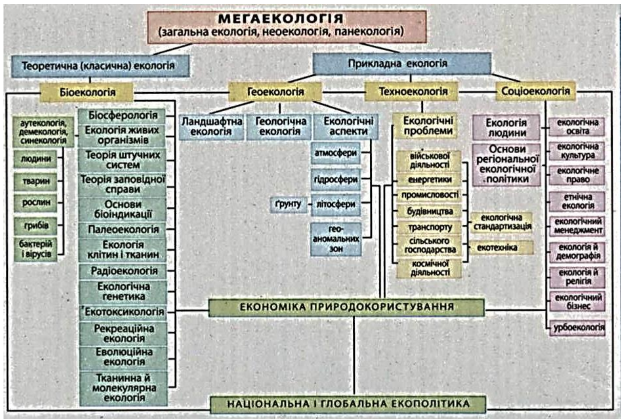
Мал.1. Структура сучасної екології
