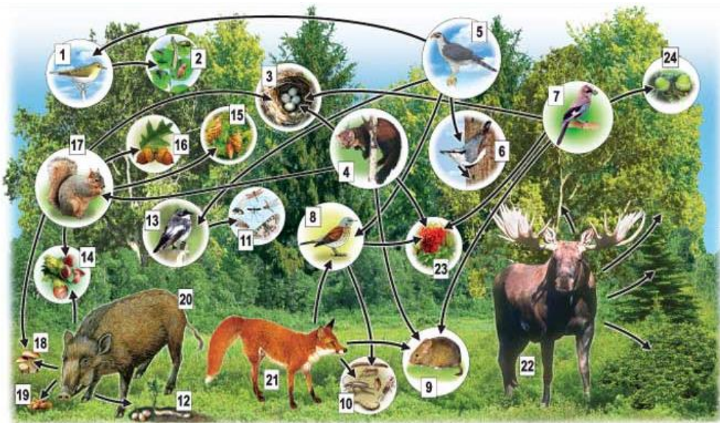
Мал.12. Трофічні зв'язки біоценозу лісу.
