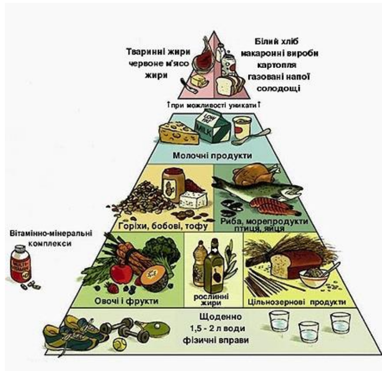
Мал.15. Додова піраміда харчування
