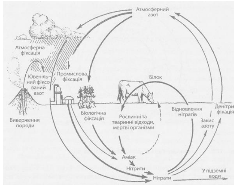
Мал.6. Кругообіг нітрогену.
