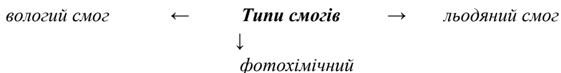
Рис. 4. Типи смогів.
