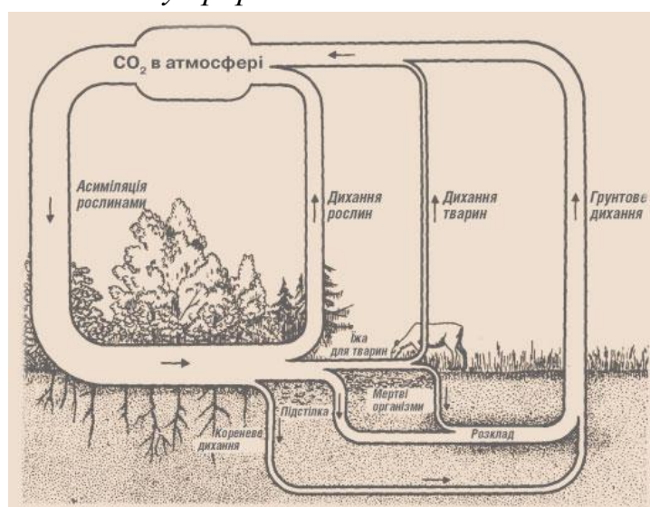
Мал. 11. Кругообіг вуглекислого газу в атмосфері.
