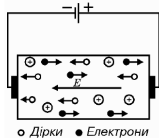
Мал. 2.13. До руху електронів і дірок у напівпровіднику під дією зовнішнього поля
