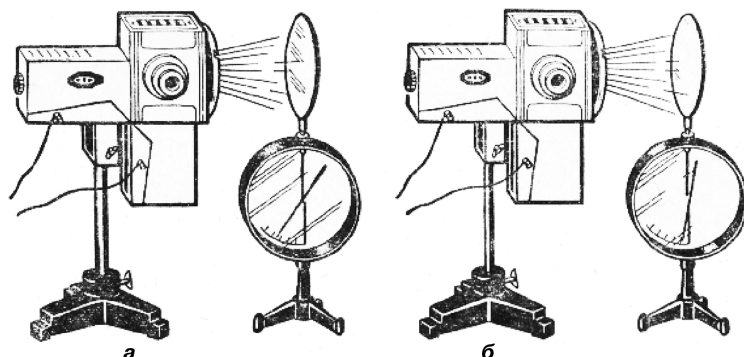
Мал. 2.44. До пояснення явища фотоелектричного ефекту
