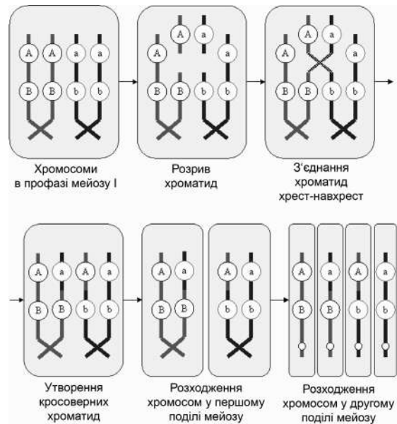
Мал. 4.14. Кросинговер
