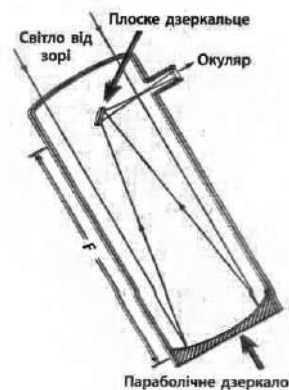
Мал. 2.64. Схема дзеркального телескопа (рефлектора)
