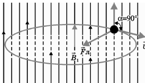
Мал. 2.17. До визначення напрямку сили Лоренца
