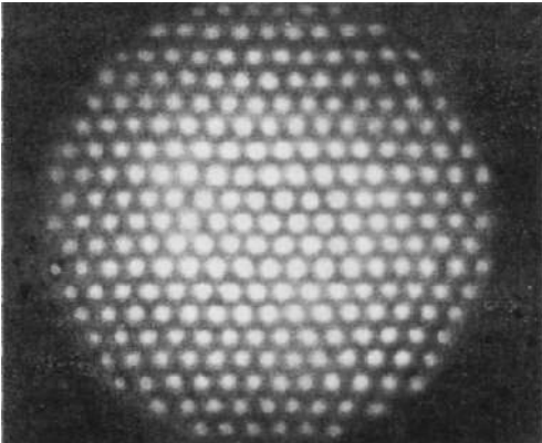
Мал. 2.48. Дифракція електронів на тонкій пластинці слюди
