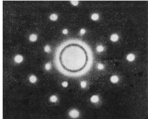
Мал. 2.49. Дифракція нейтронів на кристалі кварцу
