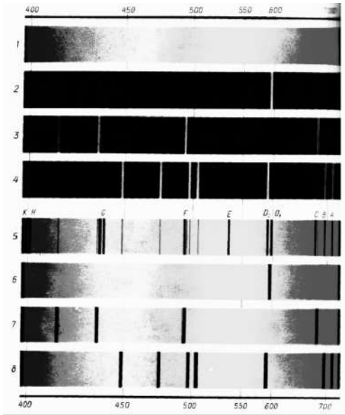
Мал. 2.53. Спектри випромінювання: 1 — суцільний, 2 — Натрію, 3 — Гідрогену, 4 — Гелію. Спектри поглинання: 5 — сонячний, 6 — Натрію, 7 — Гідрогену, 8 — Гелію
