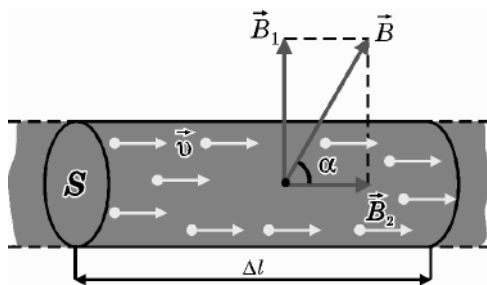
Мал. 2.16. До виводу формули сили Лоренца
