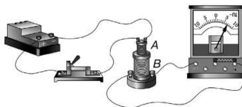
Мал. 2.19. Установка для виявлення явища електромагнітної індукції
