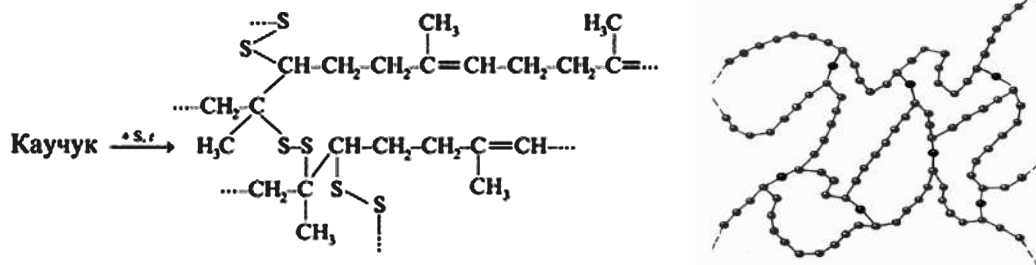
Мал. 3.19. Схема будови вулканізованого каучуку (гуми)
